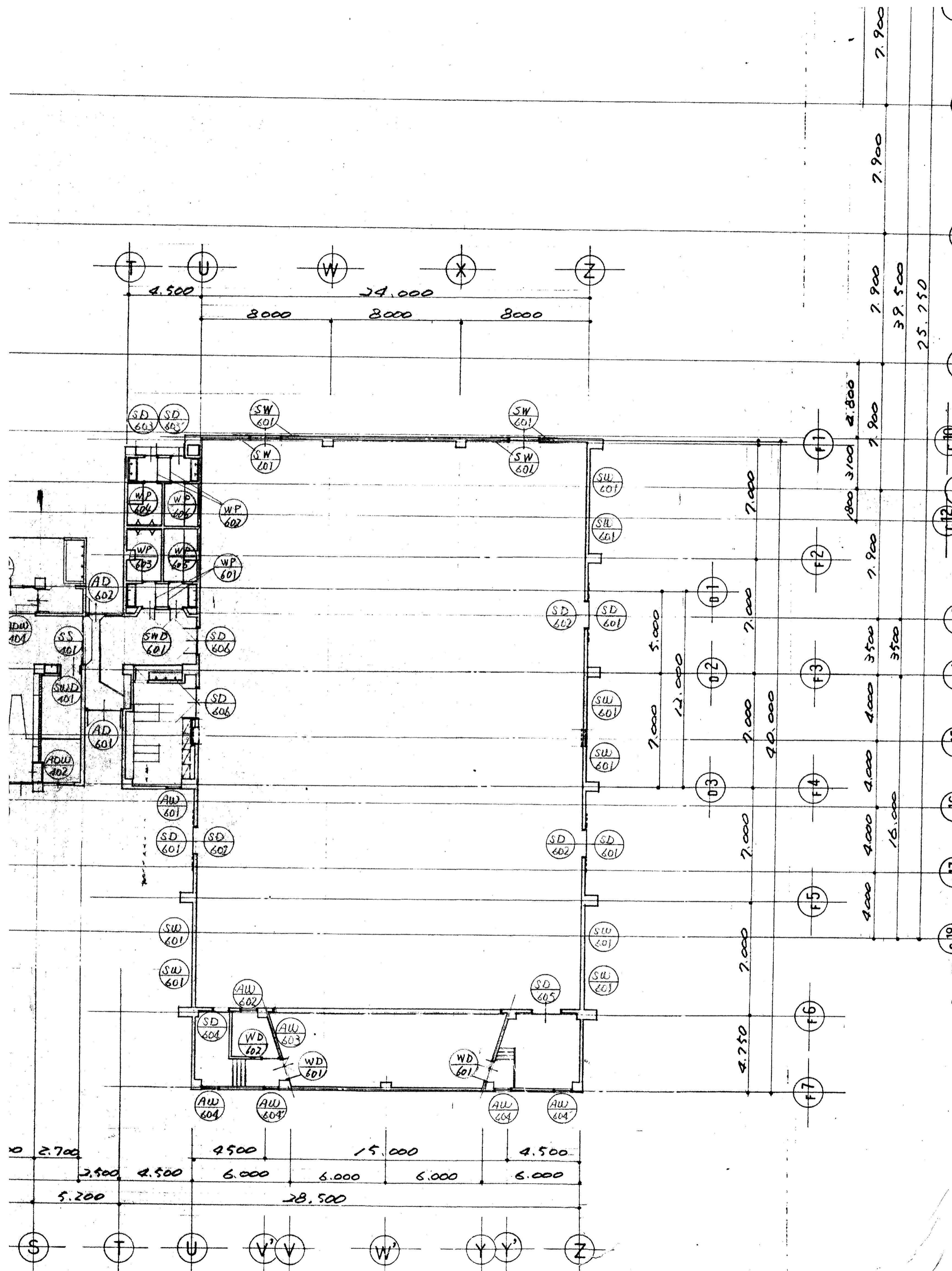
ALE MAP NAME CONSTRUCTION NAME MAP 200 1階建具指示平面図 朝日小学校改築工事 No. A-64
