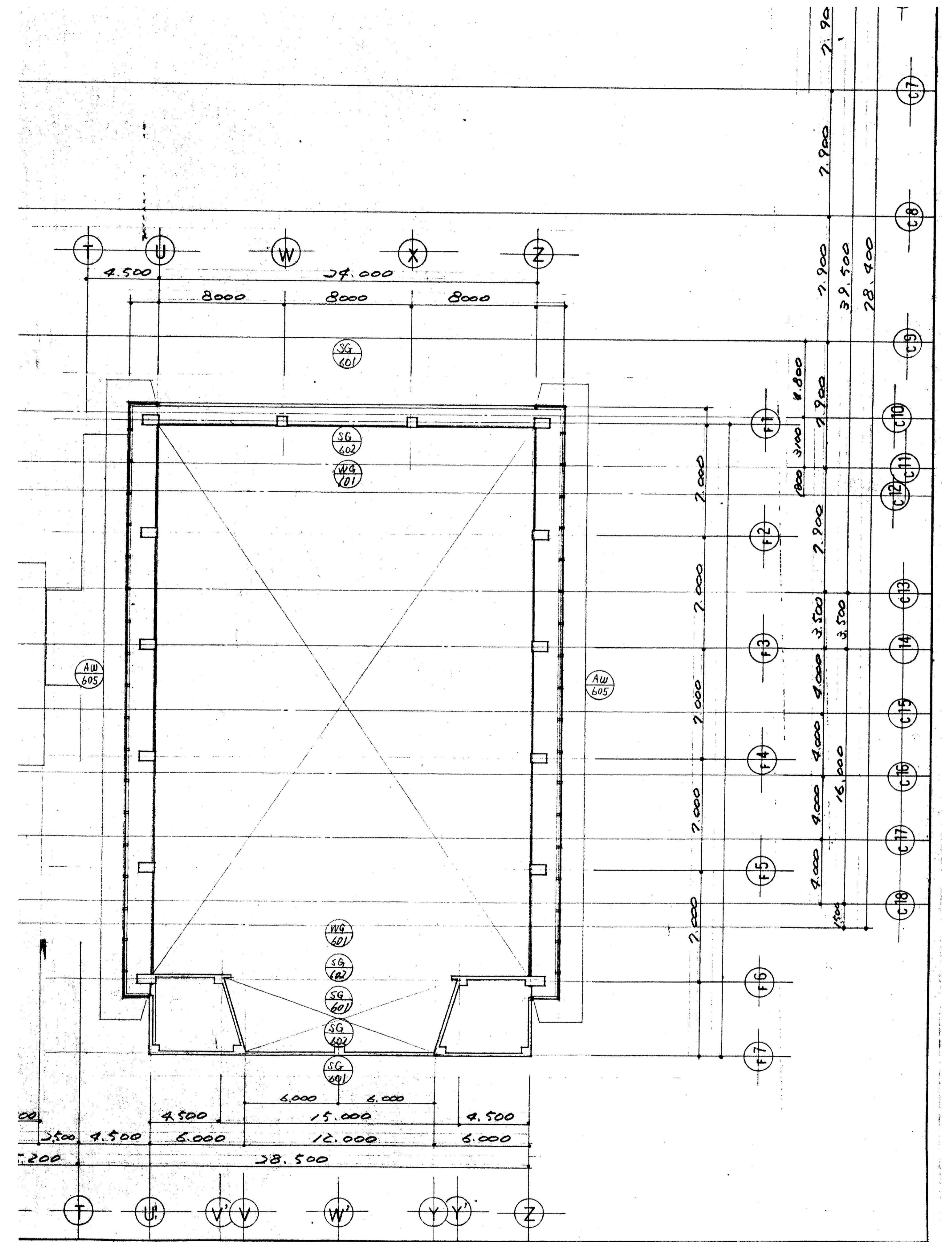
MAP NAME CONSTRUCTION NAME MAP 1階建具指示平面図 朝日小学校改築工事 No. A-65
