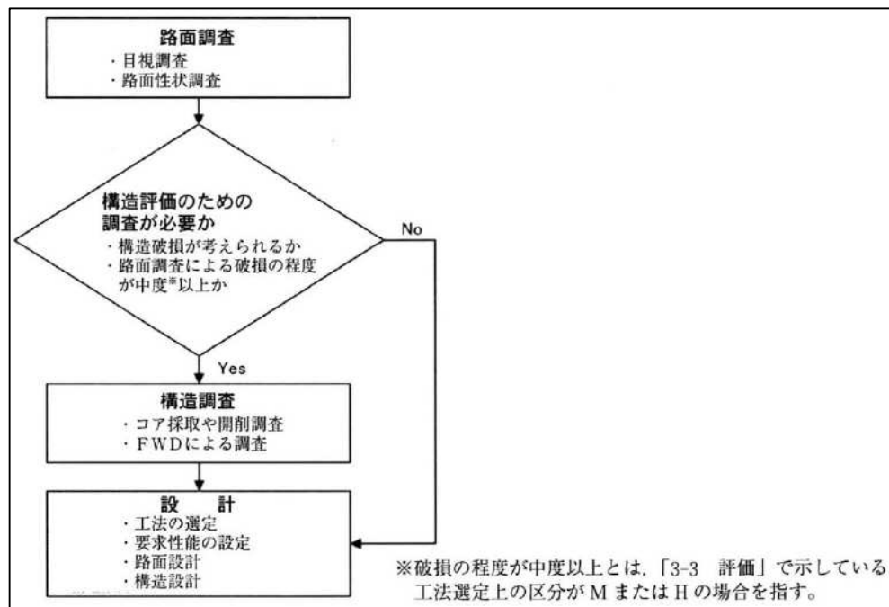
図-1.6.1.1 舗装の調査フロー
